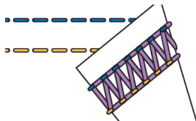
3-ниточный широкий распошивальный шов (LC- RC)
