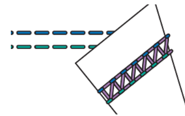
3-ниточный узкий распошивальный шов (CC- RC)
