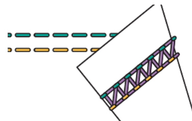
3-ниточный узкий распошивальный шов (LC- CC)
