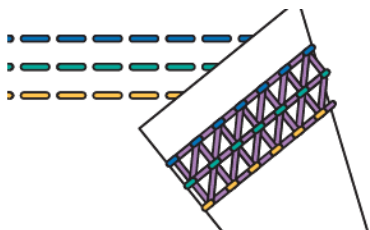
4-ниточный распошивальный шов
