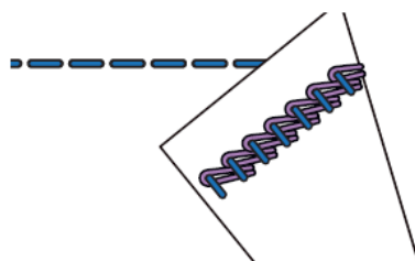
2-ниточная цепная строчка (RC)
